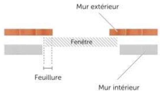
Mur plein avec feuillure (rare)
