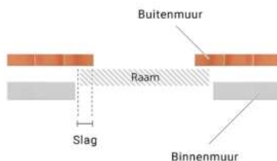
Volle muur met slag (uitzonderlijk)
