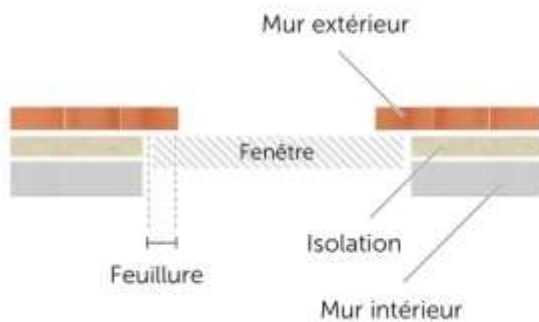
Mur creux Avec feuillure (courant)
